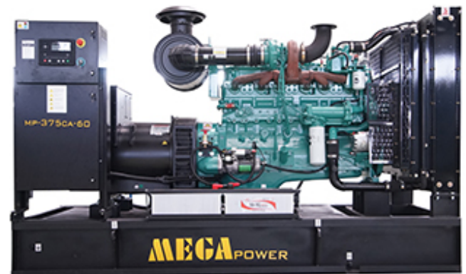
Série MP- C, propulsée par des moteurs diesel cummins : 10-3250 kva
